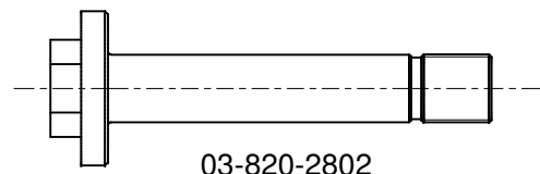
03-820-2802 Loadcell Bolt - 150 & 200kN
